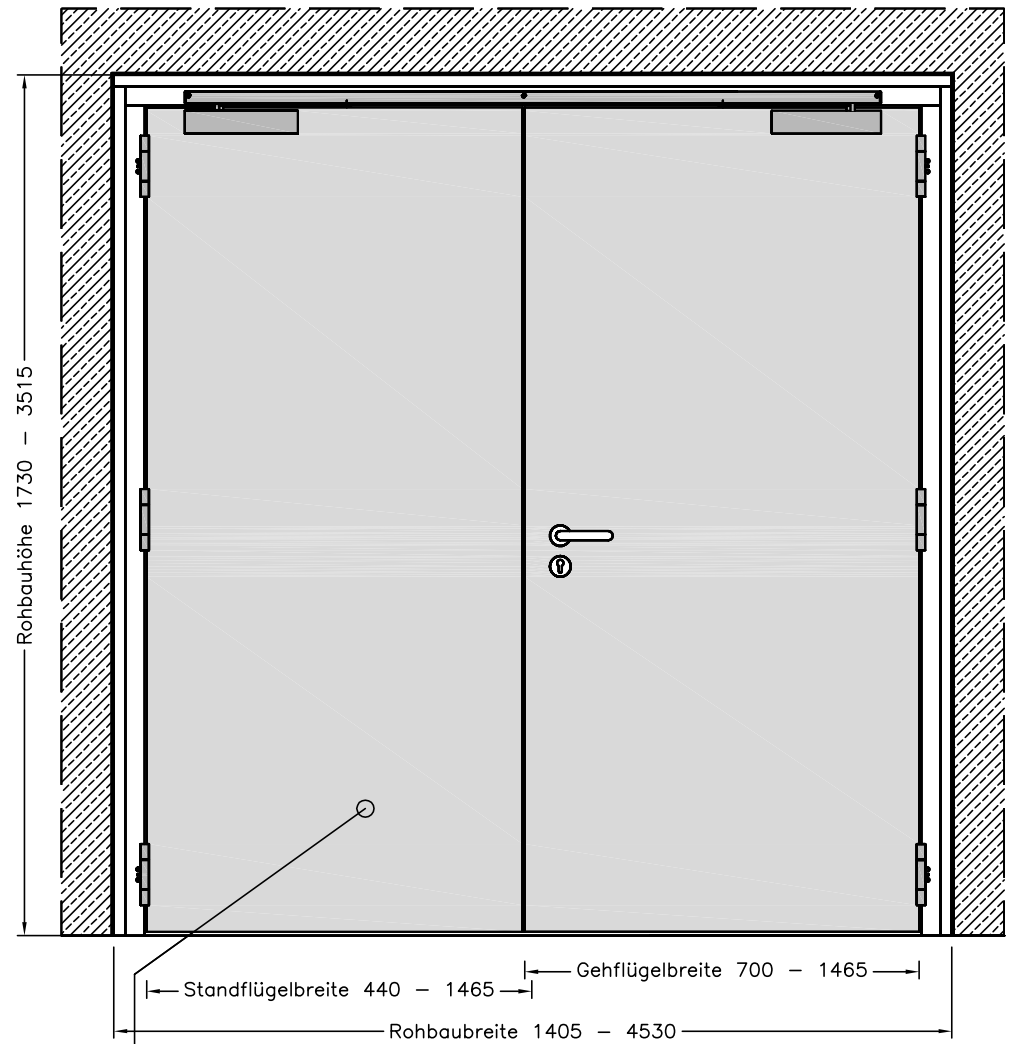
Ansicht Flurseite
