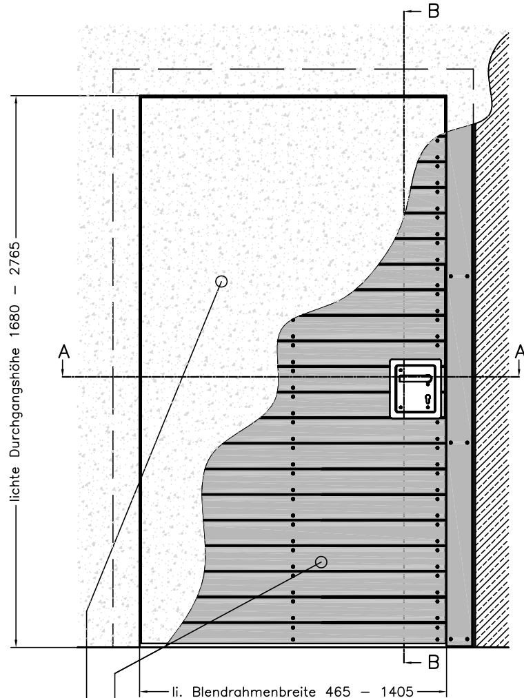
Ansicht Hallenseite
