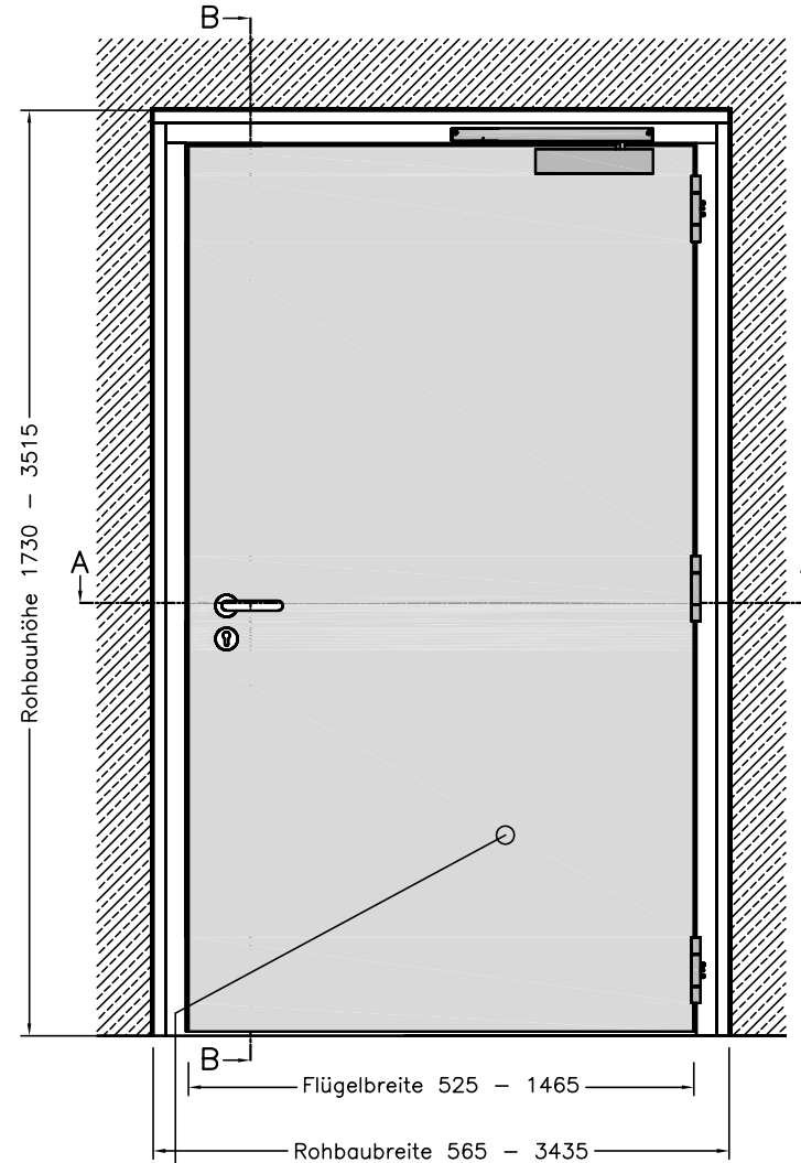
Ansicht Flurseite
