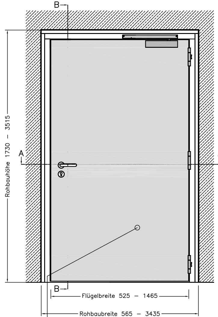
Ansicht Flurseite
