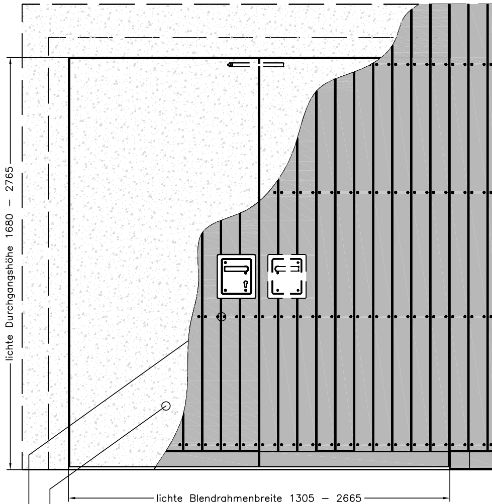
Ansicht Hallenseite
